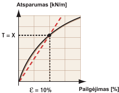
14 pav. Pradinis modulis = Kirstinės modulio, kai pvz. \epsilon = 10\%
