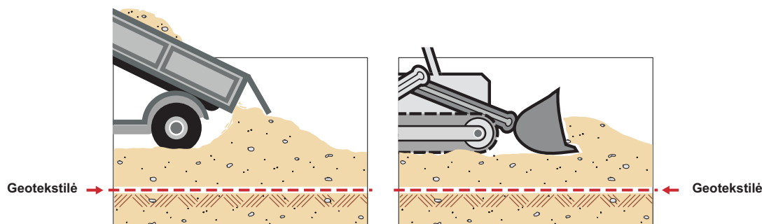
24 pav. Užpildo išpylimas neužvažiuojant ant Typar ® SF
