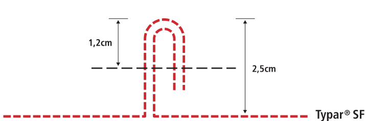
44 pav.: Rekomenduojama siūlė.
