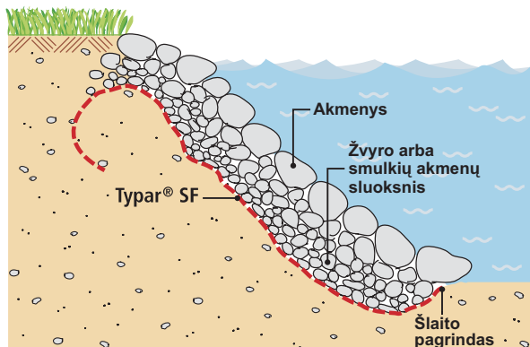
39 pav. Typar® SF pritaikymas apsaugai nuo erozijos.
